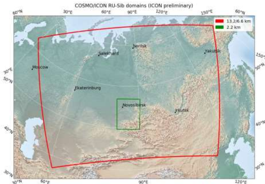
Рисунок 1 – Области оперативного прогноза системы COSMO-RU-SIB
