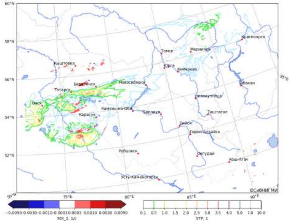
Рисунок 13 – Поле индекса обнаружения суперячеек SDI и показателя риска формирования значительных смерчей STP (16 UTC 25.06.2022)
