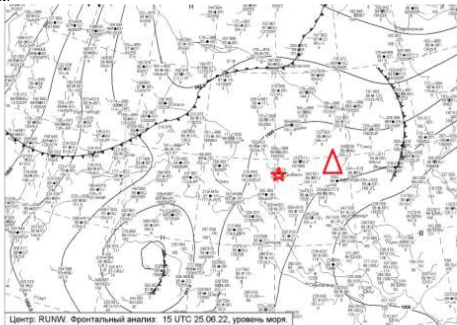
Рисунок 3 – Кольцевая карта за 15 UTC 25.06.22
