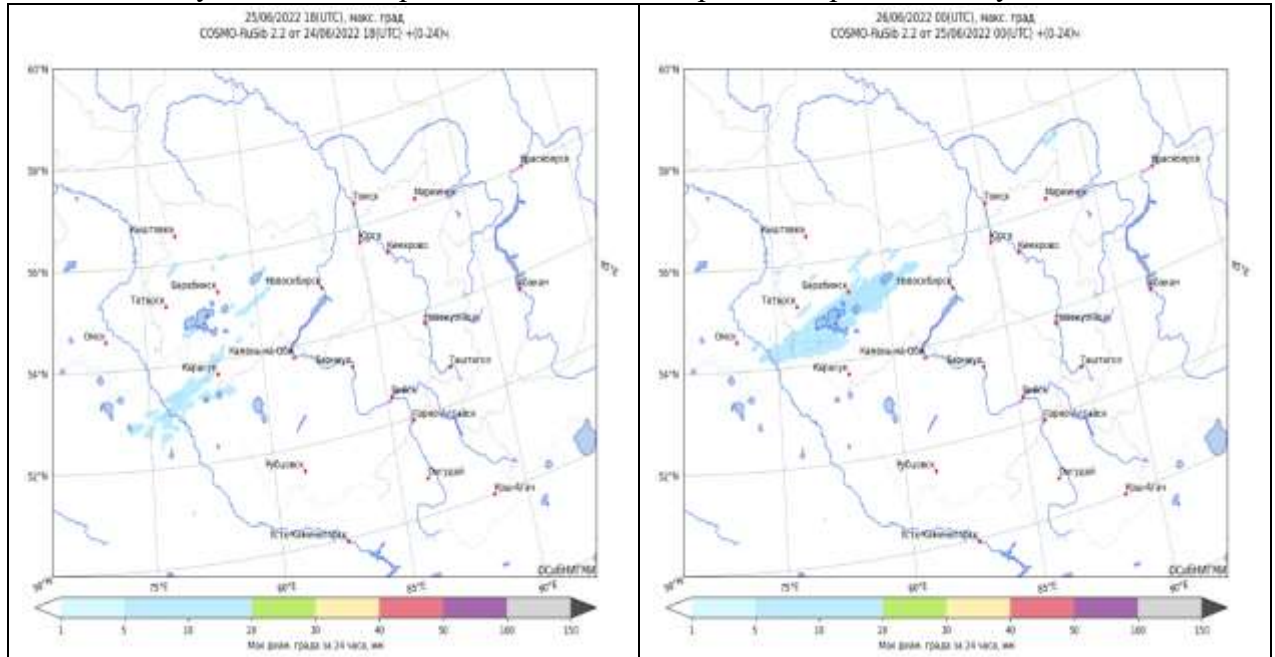
Рисунок 14 – Поле максимального диаметра градин на 24 часа для прогноза от 18 UTC 24.06.2022 (слева) и от 00 UTC 25.06.2022 (справа)
