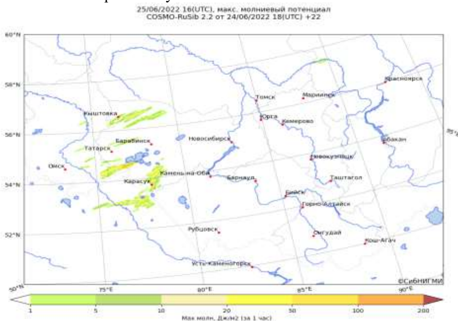
Рисунок 12 – Поле максимального молниевоего потенциала LPI (16 UTC 25.06.2022)
