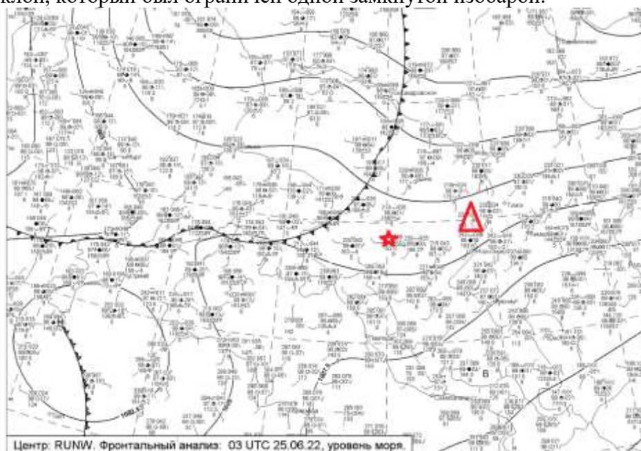
Рисунок 2 – Кольцевая карта за 03 UTC 25.06.22
