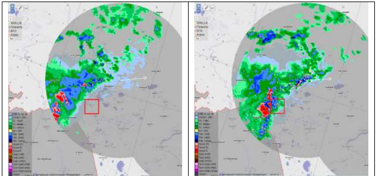
Рисунок 8 – Обзоры ДМРЛ за 14:00 и 15:00 UTC (слева и справа соответственно)
