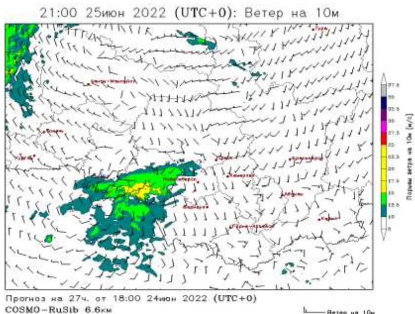
Рисунок 17 - Поле скорости, направления и порыва ветра COSMO-Ru-SIB 6.6 (21 UTC 25.06.2022)
