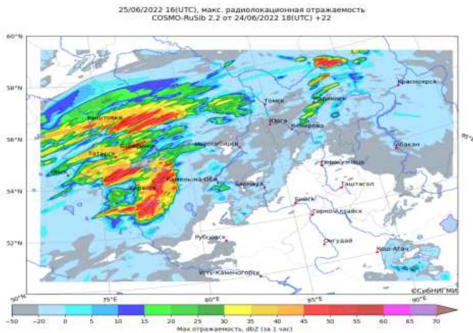
Рисунок 11 – Поле радиолокационной отражаемости (16 UTC 25.06.2022)
