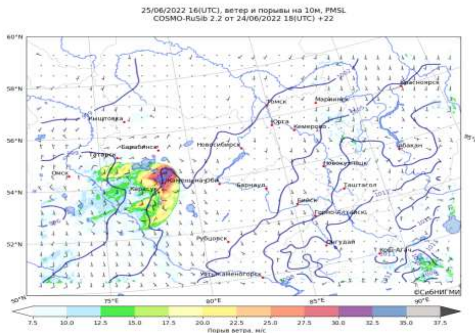
Рисунок 15 – Поле скорости, направления и порыва ветра (16 UTC 25.06.2022)
