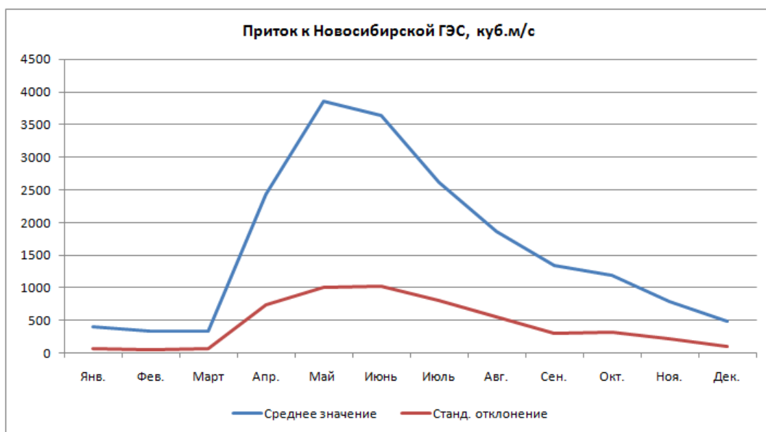
Рисунок 17 - Сезонная изменчивость среднего многолетнего значения и стандартного отклонения притока к Новосибирской ГЭС
