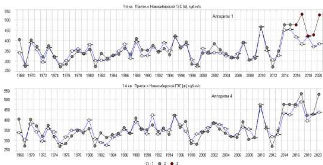
Рисунок 22 - Аппроксимация и прогноз притока в 1-м квартале по моделям, построенным по алгоритмам 1 и 4. Обозначения: 1 – математическое ожидание модельной оценки, 2,3 - фактические значения (2 – обучающая выборка, 3 – контрольная выборка)
